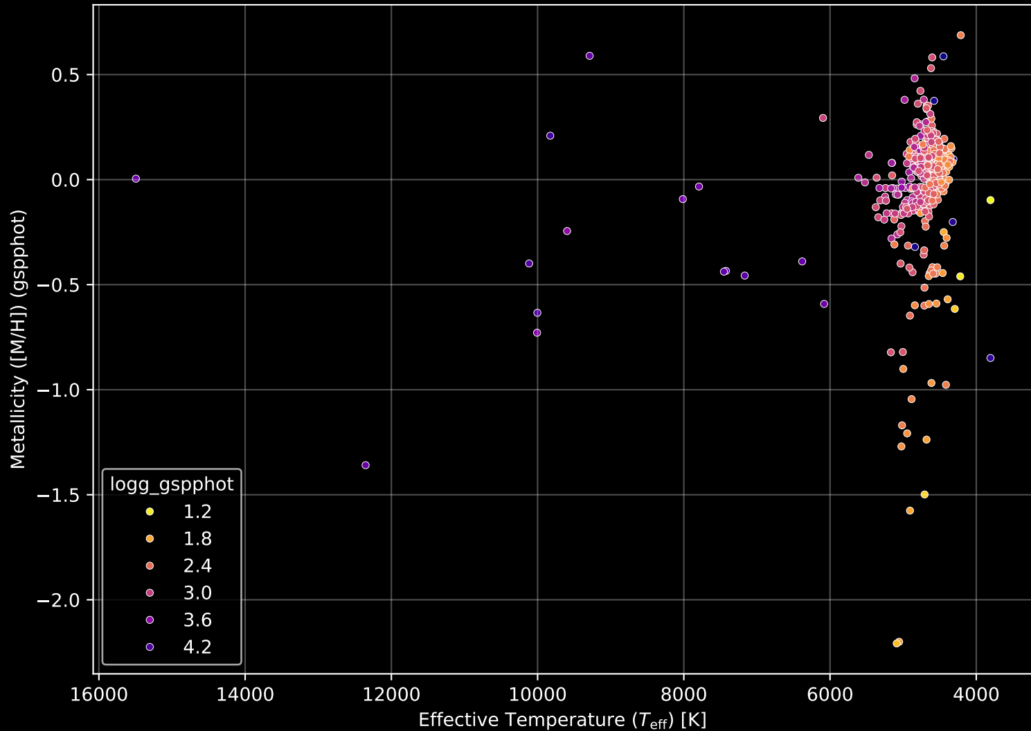
APOGEE DR17 Field: [064+06] Stellar Population Parameters (n= 430)
